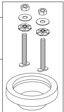
RP100491 Mounting Hardware Herraje para la instalación Pièces de montage
