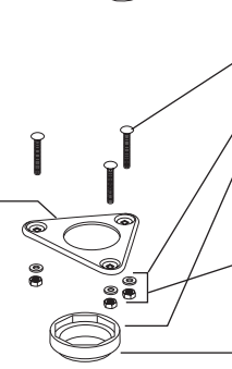
RP100493 Nuts (3), Washers (3), Bolts (3) & Seal Tuercas (3), Arandelas (3), Pernos (3), y Sello Écrous (3), rondelles (3), boulons (3) et joint d'étanchéité
