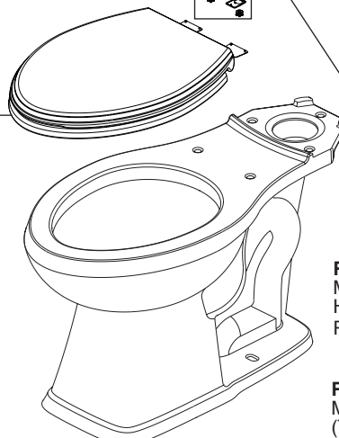
811901 ▲ Seat Assembly EL Ensamble del asiento - EL Siège - EL
